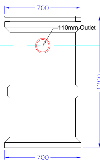
Elevation B.
