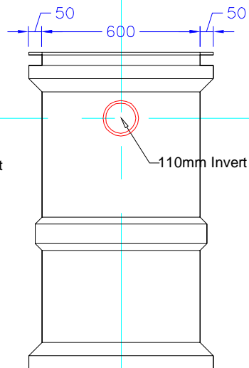
Elevation A.
