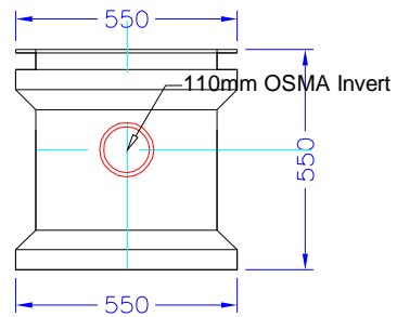
Elevation B.
