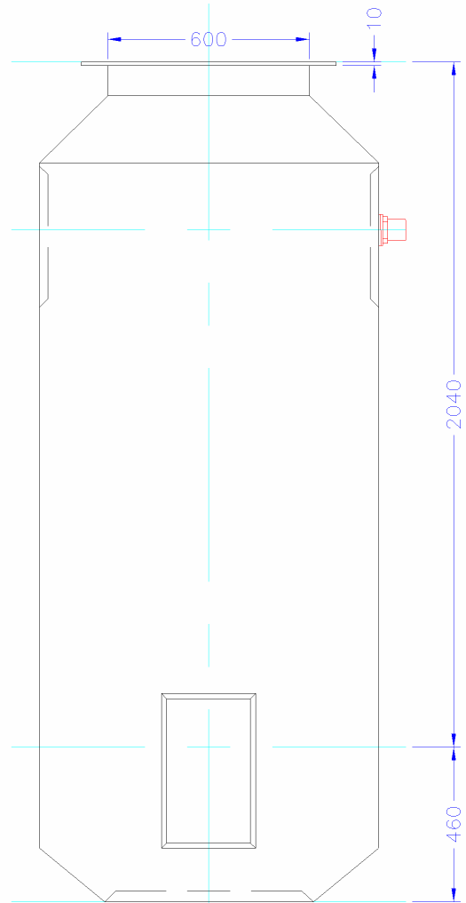
Elevation A.
