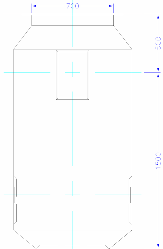
Elevation B.
